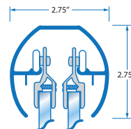
Precision Rollers
